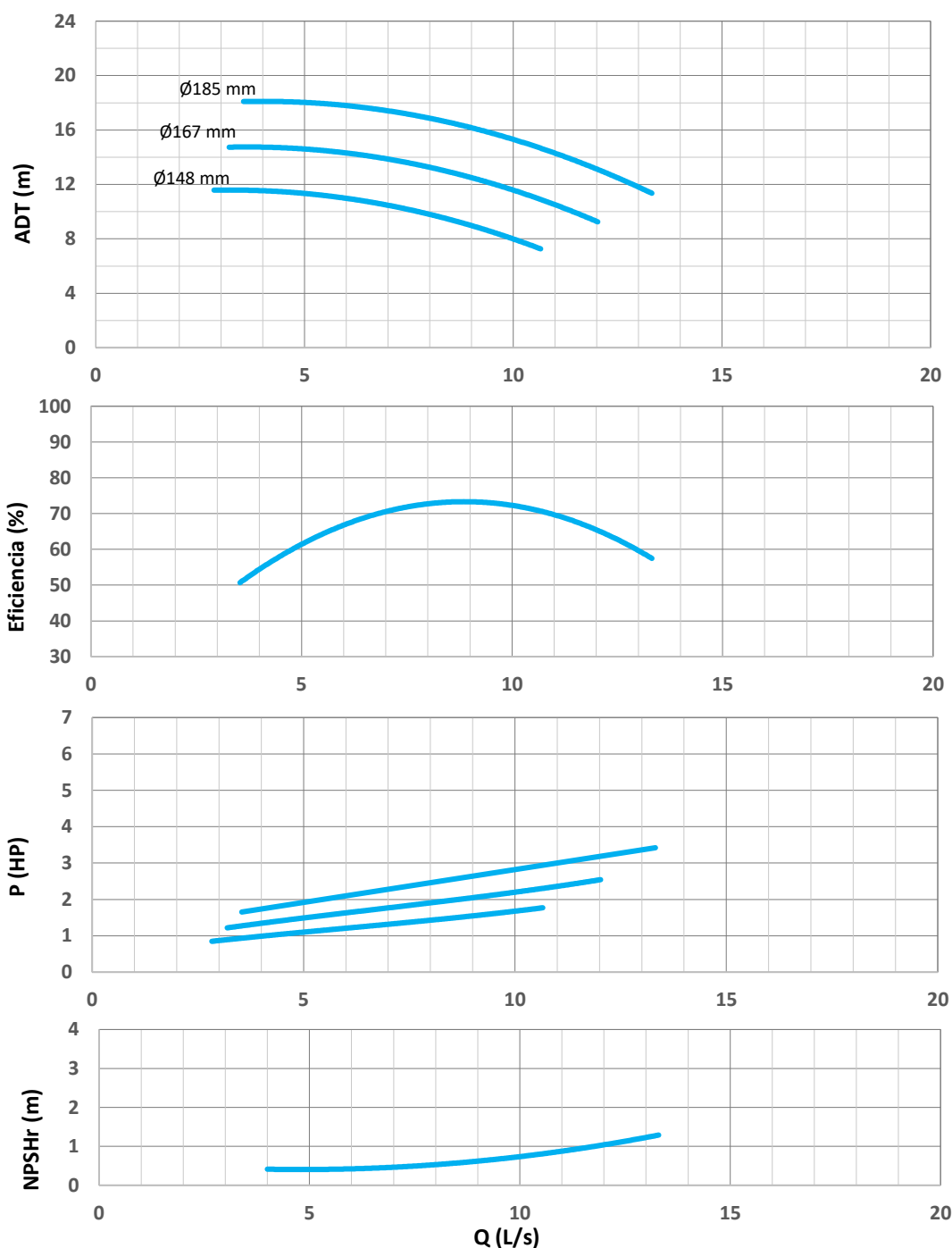
CURVAS DE OPERACIÓN SEGÚN NORMA ANSI/HI 14.6-2011 Grado 2B
